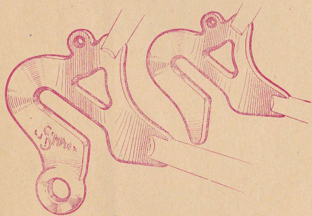
PATTES DE CADRE TYPE "JUY 543" Découpées ou Matricées
