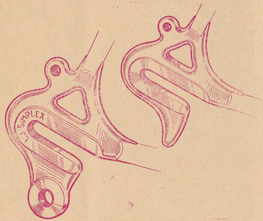
PATTES DE CADRE TYPE "JUY 543" Découpées ou Matricées
